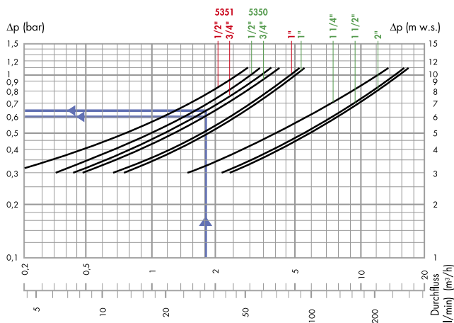
Abbildung 2 (Druckverlust)
